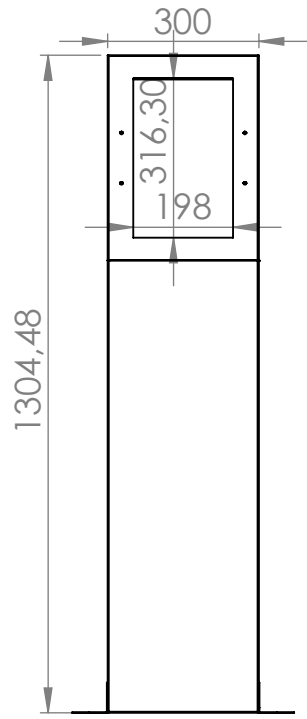
ÖN
